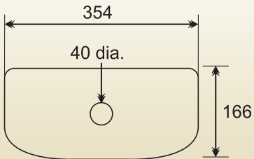
Top Elevation
